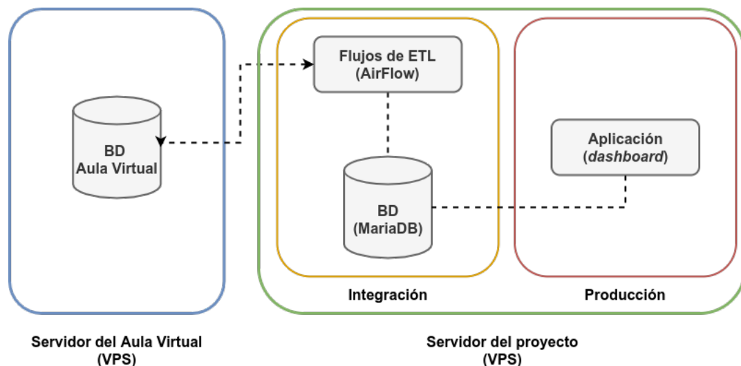
Figura 5.2: Arquitectura inicial del proyecto.
