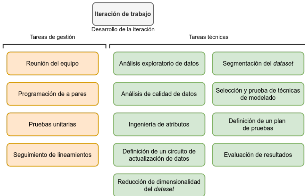
Figura 4.4: Tareas ejecutables en el desarrollo de cada iteración.
