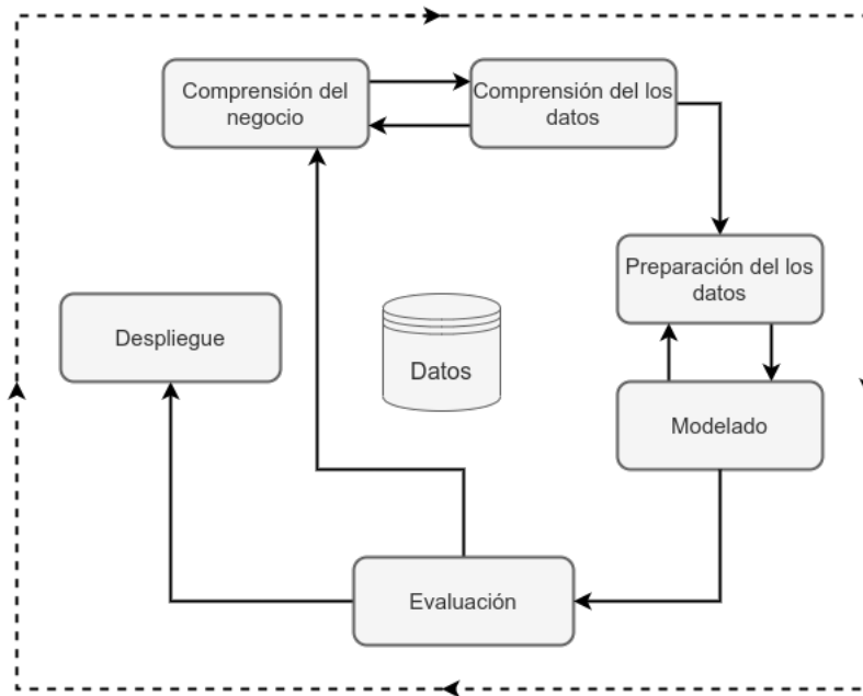
Figura 2.2: Fases del modelo de procesos CRISP-DM.
