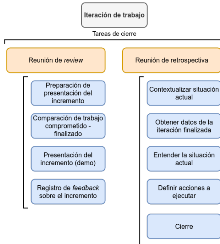
Figura 4.5: Tareas de cierre de cada iteración.
