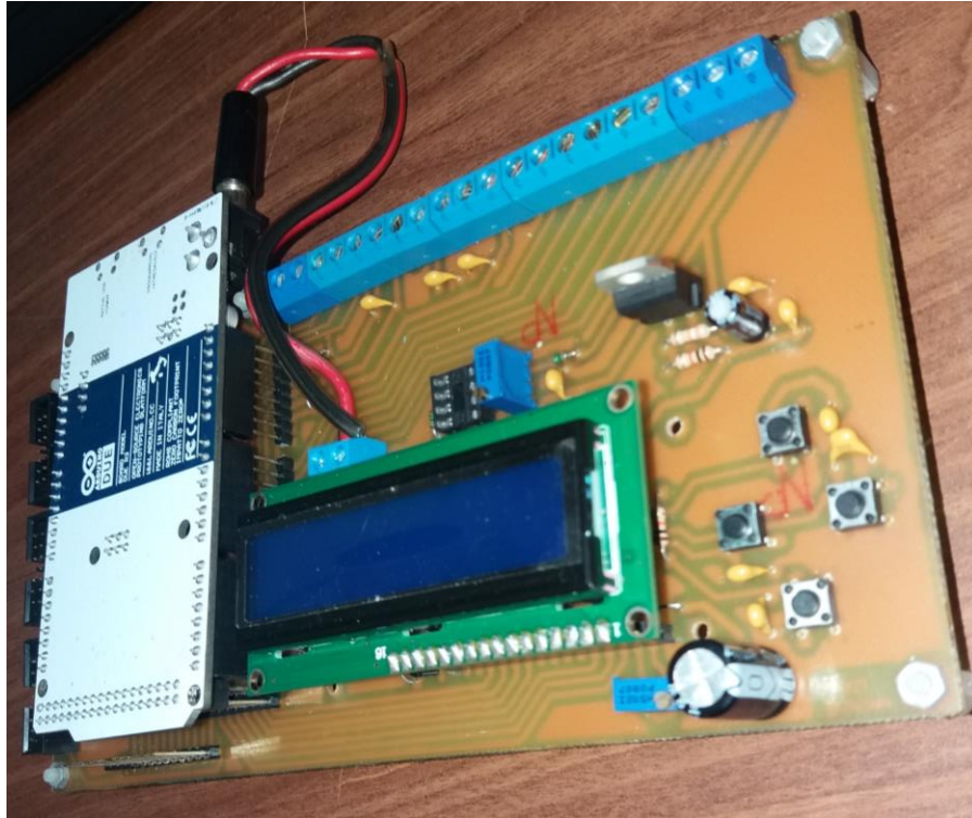
Figura 2: Prototipo del automatismo para sistemas de riego
