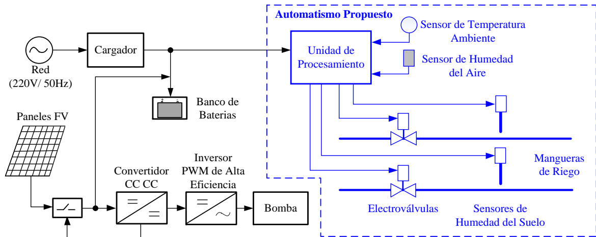
Figura 1: Automatismo propuesto en conjunto con el resto del sistema de riego
