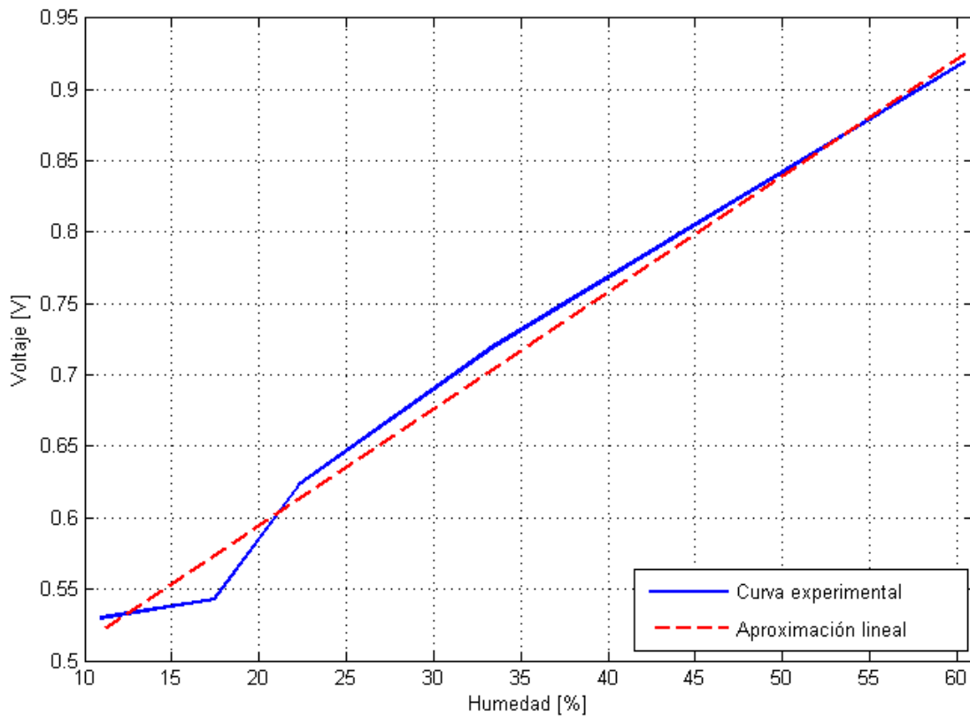
Figura 3: Curvas sensor de humedad
