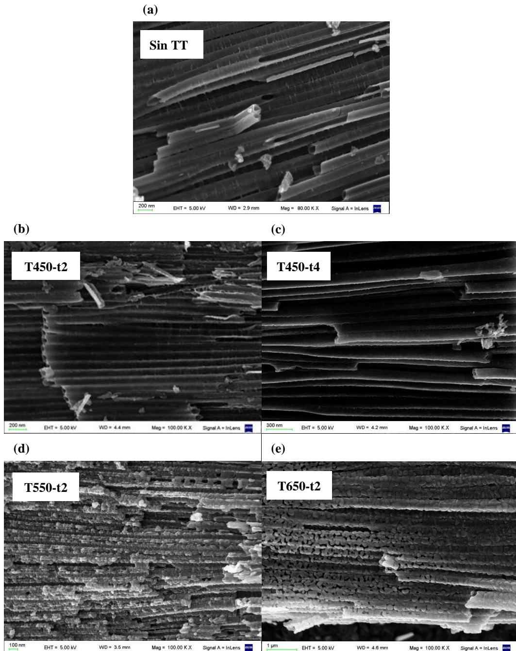
Figura 3: Micrografías electrónicas de barrido de vistas laterales de los nanotubos con diferentes tratamientos térmicos.
