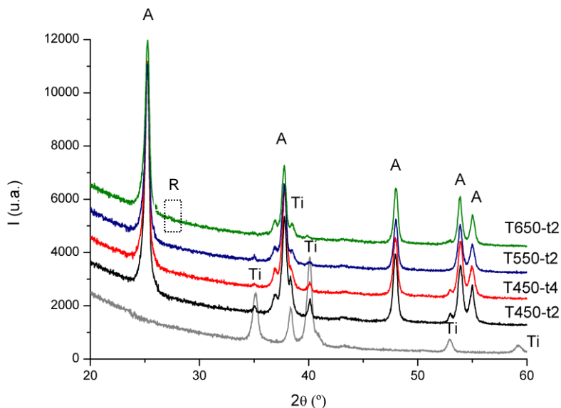
Figura 2: Difractogramas de rayos X del sustrato de Ti y de los recubrimientos estudiados. Los picos indexados con A corresponden a la fase anatasa, con R a la fase rutilo y con Ti al titanio.
