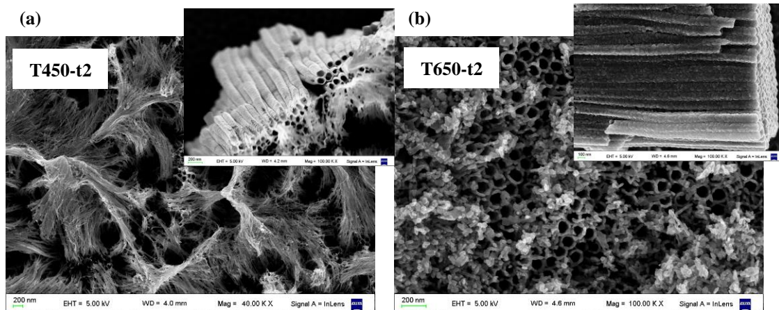
Figura 1: Micrografías electrónicas de barrido de vistas frontales y en perspectiva de los nanotubos.
