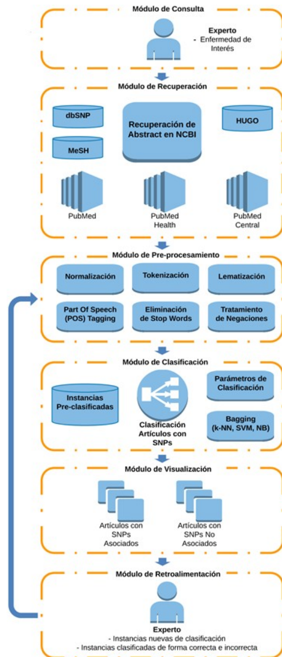
Figura 2. Esquema del Meta-estimador
