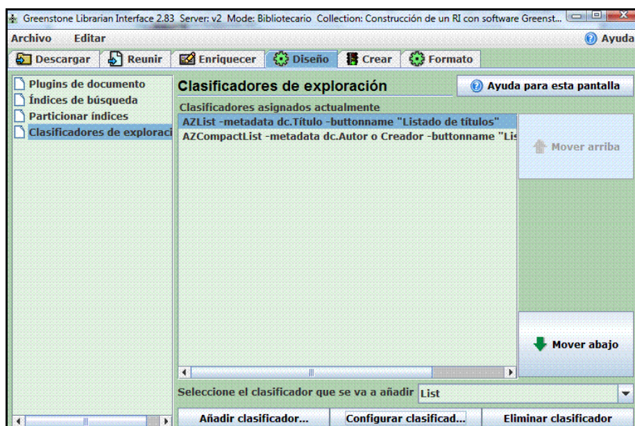
Fig. 30: Creando la colección: definición de clasificadores
