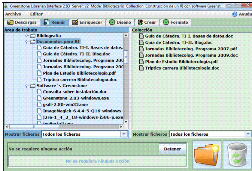
Fig. 22: Creando la colección: reuniendo los documentos
