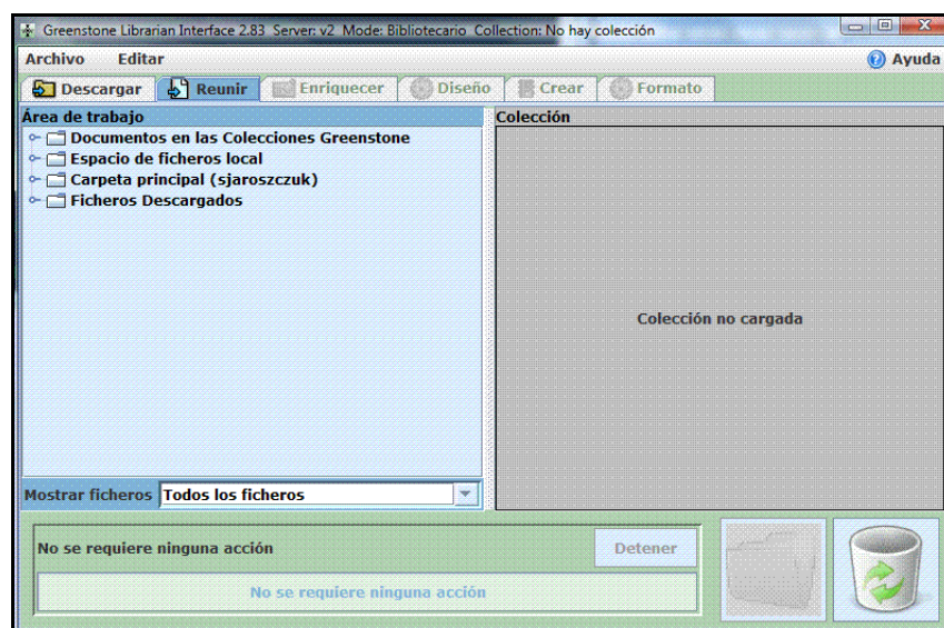
Fig. 20: Interface GLI
