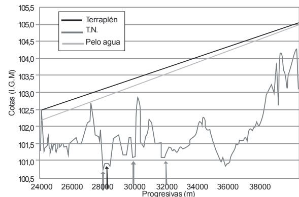
Figura 3. Altimetría de la cota de terraplén propuesto, terreno natural y cota máxima de pelo de agua.
