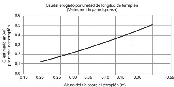
Figura 7. Curva de descarga sobre el terraplén por unidad de longitud del mismo.
