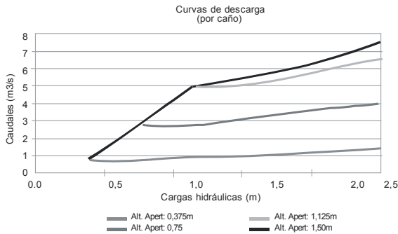
Figura 6. Curvas de descarga (por conducto).
