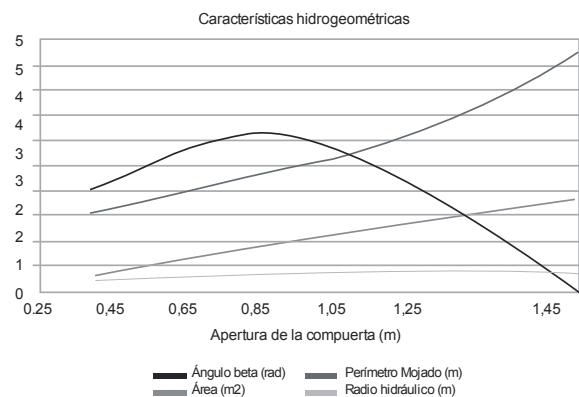
Figura 5. Características hidrogeométricas según la posición de la compuerta.
